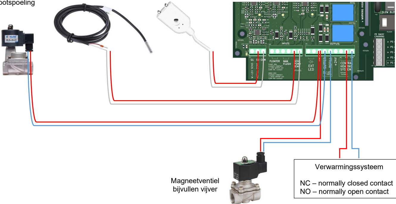
Temperatuur sensor
